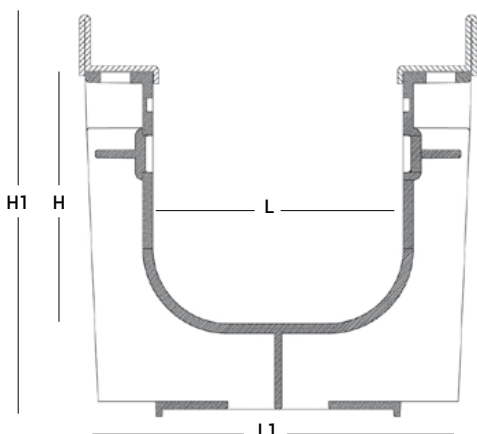
Canale PP con bordi in acciaio
