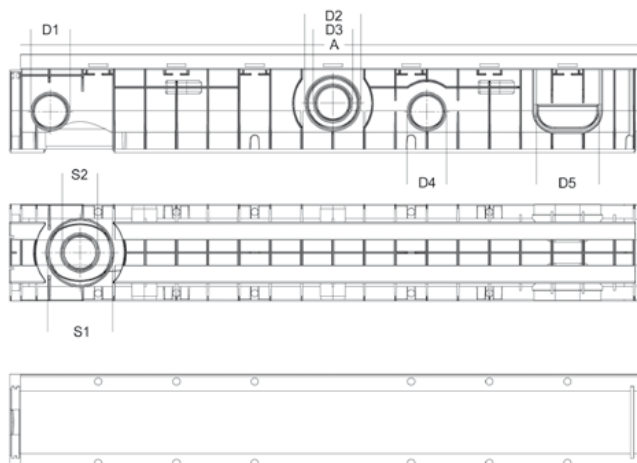
Caniveau PP bordure en acier
